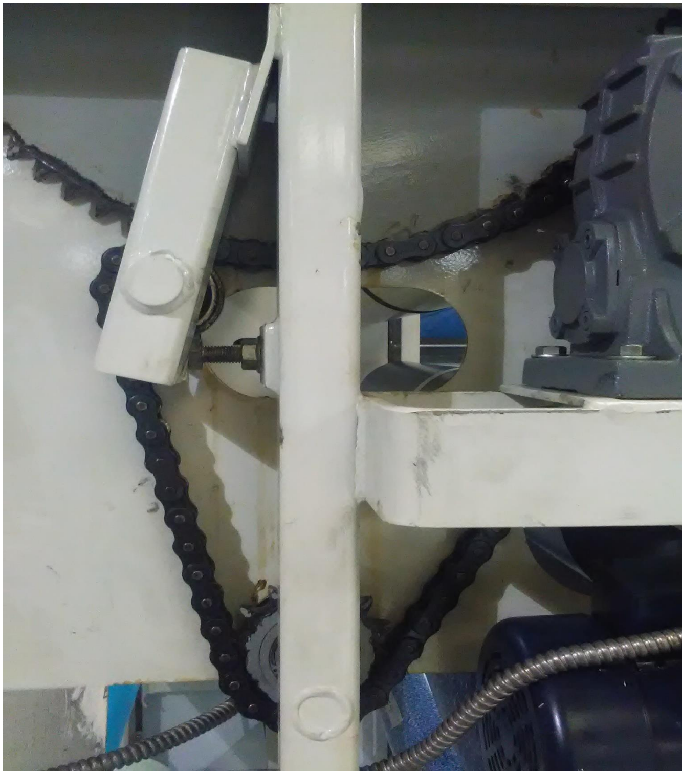
Chain Tensioner Bolt.
